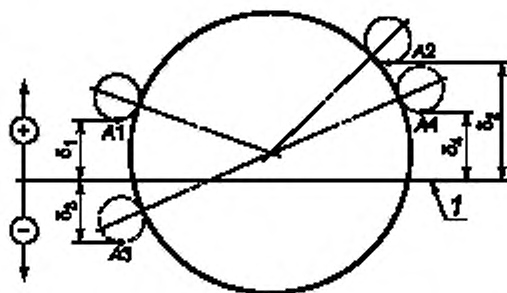
1 — линия номинального положения контрольных точек замков, наносимая на шаблон; \delta — измеряемое по вертикали отклонение замка от номинального положения; A_1, A_2 — контрольные точки первого торца; A_3, A_4 — контрольные точки второго торца; A_1, A_3 — контрольные точки первого замка; A_2, A_4 — контрольные точки второго замка
