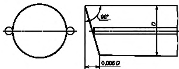
Рисунок 6 — Предельный перекосяк плоскости торца шпунтового профиля
