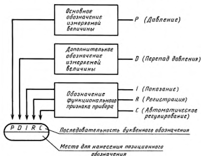
Принцип построения условного обозначения прибора
