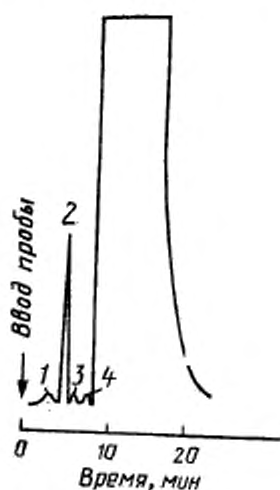
Типовая хроматограмма хлористого этила, полученная на триэтиловом эфире масляной кислоты
