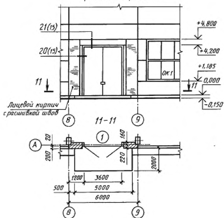
Фрагмент 3 фасада
