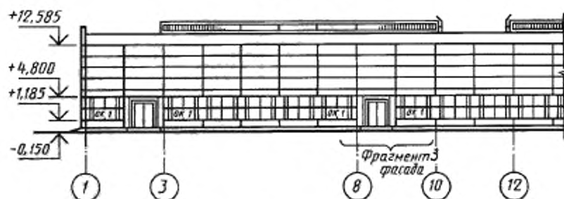
Фрагмент 3 фасада
