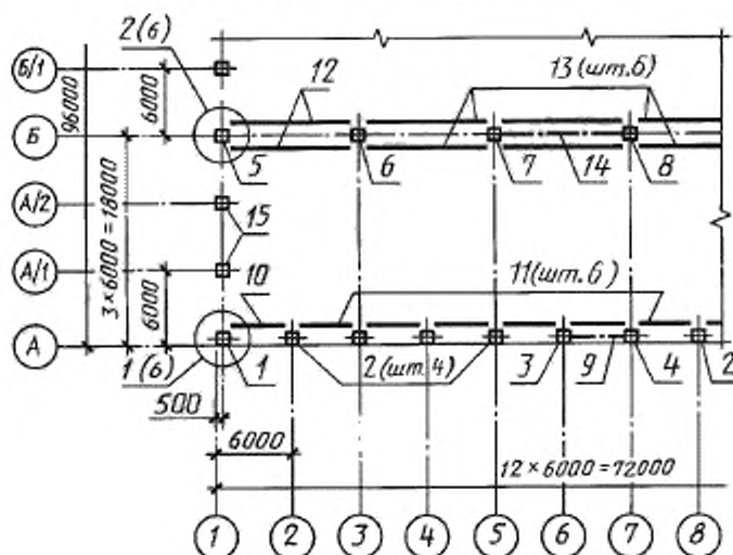
Схема расположения колонн и подкрановых балок
