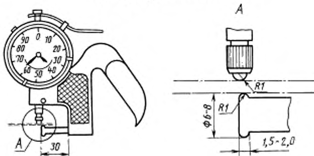
Прибор с круговой шкалой
