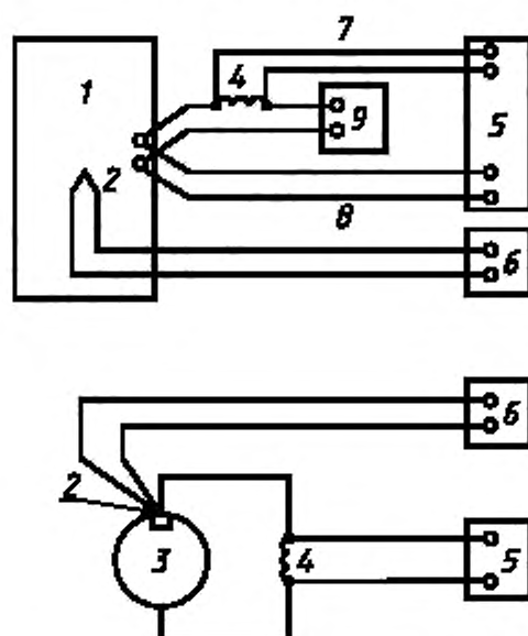
Измерительная схема
