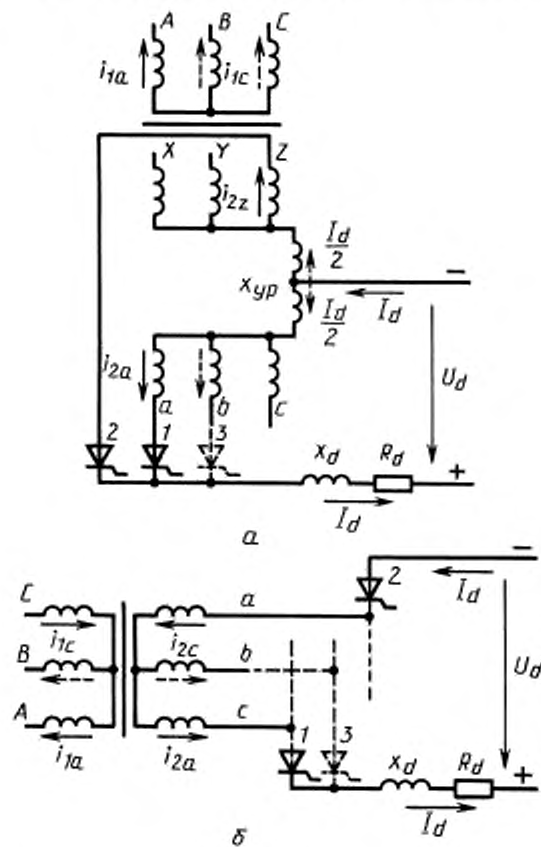
а — две обратные звезды с уравнивающим реактором; б — трехфазная мостовая
