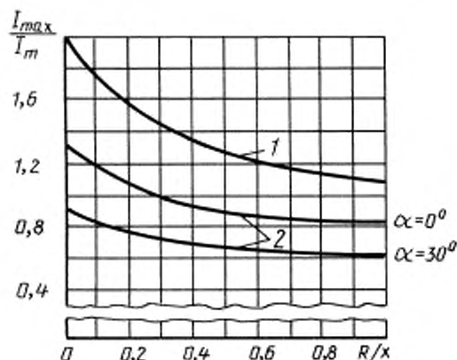
1 — неуправляемый выпрямитель; 2 — управляемый выпрямитель с электронной защитой
