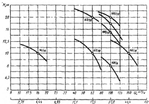
Поле Q-H
