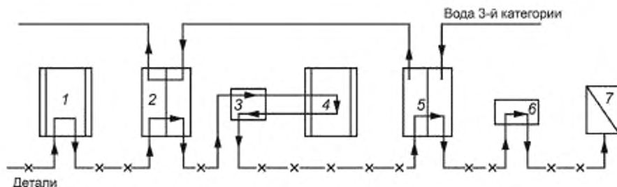
1 — ванна активации; 2, 5 — ванны промывки; 3 — ванна улавливания с водой 3-й категории; 4 — ванна нанесения покрытий; 6 — обдув сжатым воздухом или центрифугирование; 7 — сушилка (термосушка)
