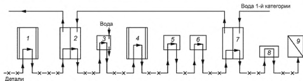
1 — ванна активации; 2, 7 — ванны промывки; 3 — ванна финишной промывки водой 3-й категории (непроточная или циркулирующая); 4 — ванна нанесения покрытий драгметаллами; 5, 6 — ванны-уловители с водой 3-й категории; 8 — обдув сжатым воздухом или центрифугирование; 9 — термосушка
