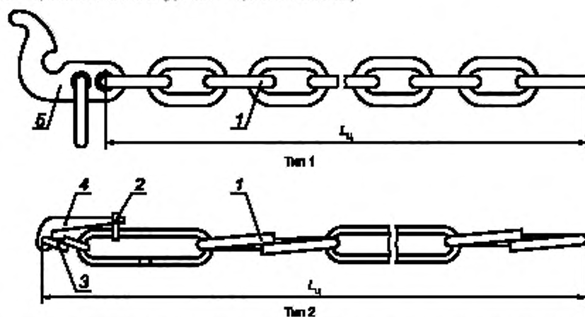
1 — цепная часть; 2 — накидное кольцо; 3 — соединительное звено; 4 — рычаг; 5 — замок типа «утка»; L_{\text{ц}} — длина цепи
