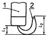
1 — корпус зажигалки; 2 — пламя
