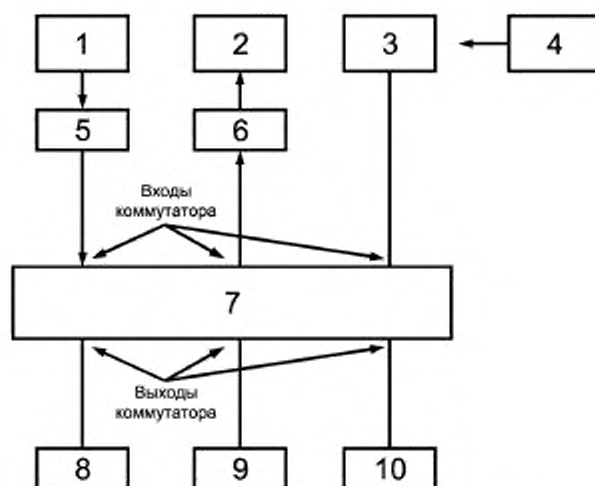
1 — генератор сигналов ВЧ; 2 — микровольтметр селективный; 3, 8, 9, 10 — согласованные нагрузки; 4 — милливольтметр ВЧ; 5, 6 — согласованные коаксиальные переходы; 7 — коммутатор
