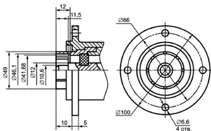
Рисунок А.1 — Присоединительные размеры несимметричных входов (выходов) коммутаторов с волновым сопротивлением 75 Ом и входной мощностью до 5 кВт
