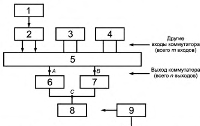
1 — генератор сигналов ВЧ; 2 — симметрирующее устройство; 3, 4 — согласованные нагрузки, 5 — коммутатор, 6, 7 — несимметричные нагрузки с волновым сопротивлением, равным половине волнового сопротивления подключаемого фидера ( W/2 ); 8 — несимметричная нагрузка с волновым сопротивлением, равным четверти волнового сопротивления подключаемого фидера ( W/4 ), 9 — милливольтметр ВЧ
