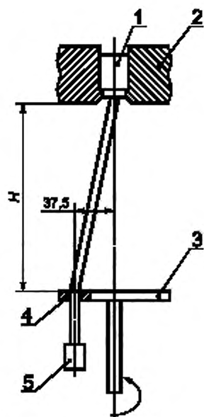
1 — зажим; 2 — оправка; 3 — плата; 4 — штупка; 5 — груз
