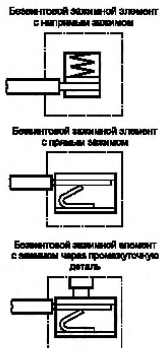
Рисунок 102 — Примеры безвинтовых зажимов
