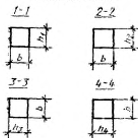
Поперечные сечения элементов ферм типоразмеров 1ФБС24...5ФБС24, 1ФБМ24...5ФБМ24
