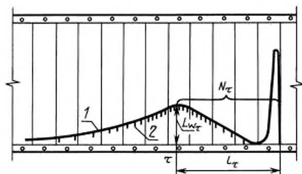
1 — кривая отклонения пера самописца; 2 — сброс пера самописца
