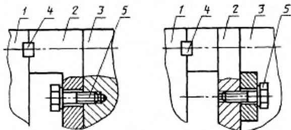
1 — МОНТАЖНАЯ ПЛТА; 2 — МОНТАЖНЫЙ МОСТИК; 3 — КОКЛЯ; 4 — ШВОНКА; 5 — БОЛТ
