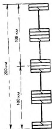
Номинальная цепь канала ТЧ местной сети
