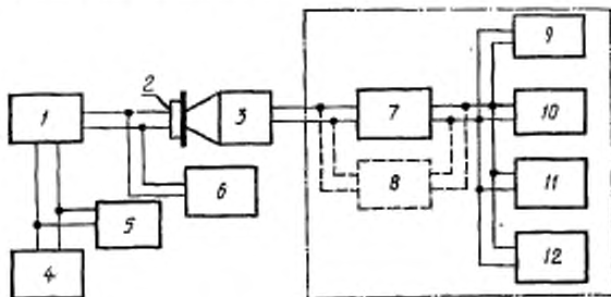
1 — аудиометр; 2 — телефон; 3 — искусственное ухо; 4 — звуковой генератор; 5 — вольтметр переменного тока; 6 — селективный микровольтметр; 7 — измерительный усилитель; 8 — селективный микровольтметр; 9 — осциллограф; 10 — частотомер; 11 — измеритель нелинейных искажений; 12 — анализатор спектра
