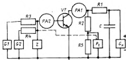
G1 —генератор однополярных насыщающих импульсов, G2 —генератор однополярных запирающих импульсов; PA1 , PA2 —импульсные измерители тока; VT —испытуемый транзистор; Z —ограничитель напряжения; R1 —резистор нагрузки; R2 , R5 —делитель напряжения; R3 , R4 —резисторы в цепи базы; Pt —измеритель интервалов времени; C —блокировочный конденсатор, Gk —источник постоянного напряжения коллектора
