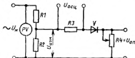
R_1, R_2, R_3 —безындукционные резисторы. R_4 —резистор; V —диод; U_n —номинальное напряжение; U_{изм} —измеряемое напряжение; U_{оп} —постоянное опорное напряжение; U_{осц} —амплитудное значение напряжения на входе осциллографа ( U_{max} > U_{оп} ); PV —вольтметр
