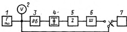
1—генератор; 2—вольтметр; 3—магазин затуханий; 4—согласующее звено; 5—эквивалент микрофона; 6—электрическая часть шумомера; 7—измеритель нелинейных искажений
