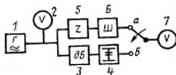
1—генератор; 2—вольтметр; 3—магазин затухания; 4—согласующее звено; 5—эквивалент микрофона; 6—электрическая часть шумомера; 7—вольтметр или самописец.
