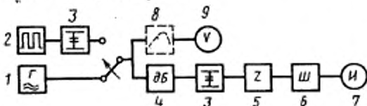
1—генератор синусоидального напряжения; 2—генератор импульсов; 3—согласующее алено; 4—магазин затуханий; 5—эквивалент микрофона; 6—электрическая часть шумомера; 7—измерительный прибор шумомера; 8—фильтр А, В, С, D по ГОСТ 17187—81; 9—вольтметр эффективных значений.
