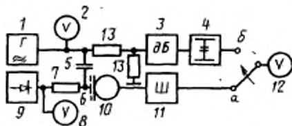
1—генератор; 2, 5—вольтметры; 3—магазин затуханий; 4—согласующее звено; 5—разделительный конденсатор; 6—электростатический возбуждатель; 7—резистор; 8—источник поляризующего напряжения; 9—источник поляризующего напряжения; 10—микрофон шумомера; 11—электрическая часть шумомера; 12—вольтметр или самописец; 13—делитель напряжения
