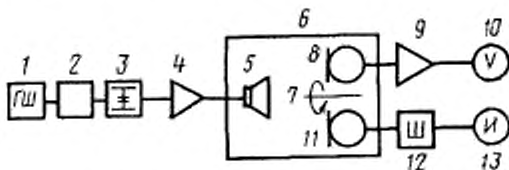
1—генератор; 2—третьоктавный фильтр; 3—согласующее звено; 4—усилитель мощности; 5—громкоговоритель; 6—реверберационная камера; 7—координатное устройство; 8—образцовый микрофон; 9—микрофонный усилитель; 10—вольтметр; 11—микрофон шумомера; 12—электрическая часть шумомера; 13—измерительный прибор шумомера
