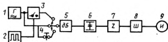
1—генератор синусоидального напряжения; 2—генератор импульсов; 3—электронный ключ; 4—механический ключ; 5—магазин затуханий; 6—согласующее звено; 7—эквивалент микрофона; 8—электрическая часть шумомера; 9—измерительный прибор шумомера
