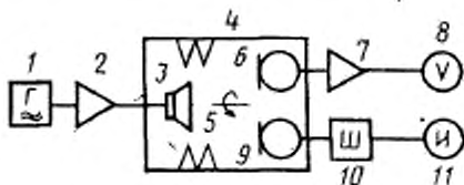
1—генератор; 2—усилитель мощности; 3—громкоговоритель; 4—заглушенная камера; 5—координатное устройство; 6—образцовый микрофон; 7—микрофонный усилитель; 8—вольтметр; 9—микрофон шумомера; 10—электрическая часть шумомера; 11—измерительный прибор шумомера
