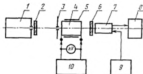
1—источник модулированного света; 2, 6—ослабители; 3—диафрагма; 4—испытуемый ЭОП; 5—держатель ЭОП; 7—приемник излучения, 8—электронно-лучевой осциллограф; 9—блок питания приемника излучения, 10—источник питания
