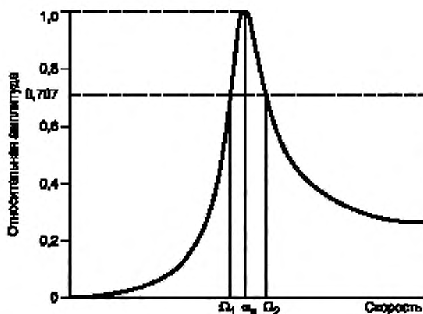
Рисунок 5 — Диаграмма Бодe для оценки модальной чувствительности
