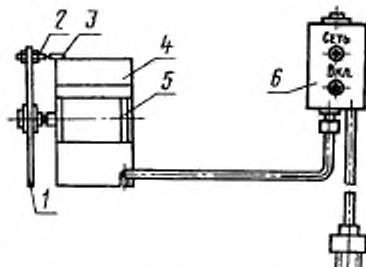
1—вращающийся диск; 2—штырек; 3—микрореле-переключатель; 4—корпус затвора; 5—двигатель; 6—пульт управления
