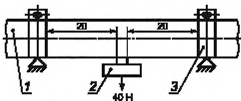
1 — пластмассовый трубопровод; 2 — разбрызгиватель; 3 — хомут
