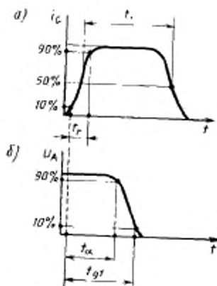
а—форма импульса тока управления тиристора; б—форма импульса анодного напряжения.
