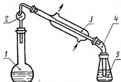
1 — колба Кьельдаля; 2 — напласовка; 3 — холодильник; 4 — аллонж; 5 — приемная колба.
