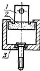
1—испытательная головка; 2—образец; 3—захват.
