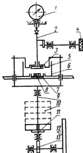
1—индикатор; 2—измерительная ось; 3—основание измерительной оси; 4—маховичок для перемещения измерительной оси; 5—матрица с электрообогревом; 6—неподвижная матрица с электрообогревом; 7—стол; 8—испытуемый образец; 9—грузовая тяга; 10—грузы; 11—площадка для грузов; 12—рукоятка; 13—эксцентрик.
