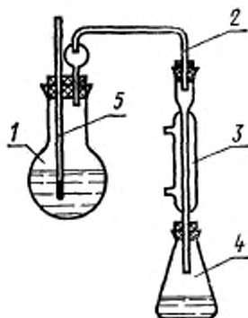
1—перегонная колба вместимостью 500 мл; 2—насадка с брызгоуловителем; 3—холодильник; 4—приемник; 5—термометр.
