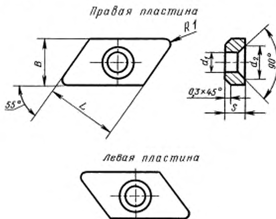
Размеры, мм
