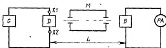
G —генератор тока; D —излучатель (проверяемый или образцовый); X1 , X2 —контакты подключения излучателя; M —спектральный прибор; B —фотоприемник; PA —измеритель тока; L —расстояние от излучателя до фотоприемника
