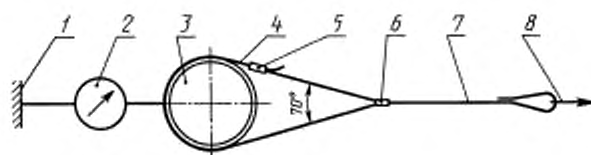
Рисунок 7 — Схема испытания пояса в целом статической нагрузкой
