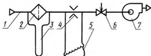
1 — воздуховоды; 2 — испытуемый фильтр-поглотитель; 3 — U-образный мановакуумметр; 4 — измерительная диафрагма; 5 — жидкостный микроманометр; 6 — регулирующее устройство; 7 — вентилятор или другой побудитель воздушного потока
