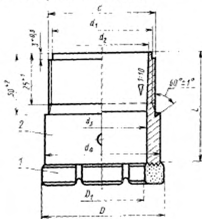
1—матрица; 2—корона.
