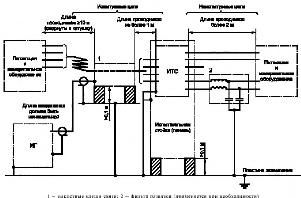
Рисунок 2 — Пример рабочего места для испытаний с применением емкостных клещей связи
