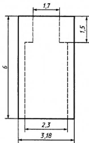
Рисунок R.1 — Кожух датчика
