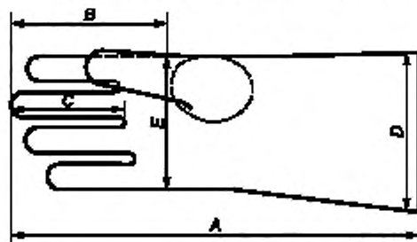
Рисунок 1 — Внутренние размеры ЗАЩИТНЫХ ПЕРЧАТОК
