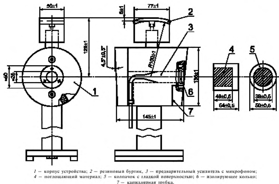
Рисунок 1 — Образец устройства для проведения акустического испытания
