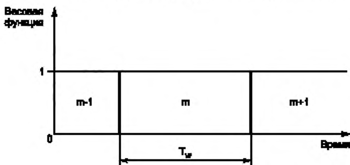
m-1 , m , m+1 — последовательность измерительных окон; T_w — ширина измерительного окна
