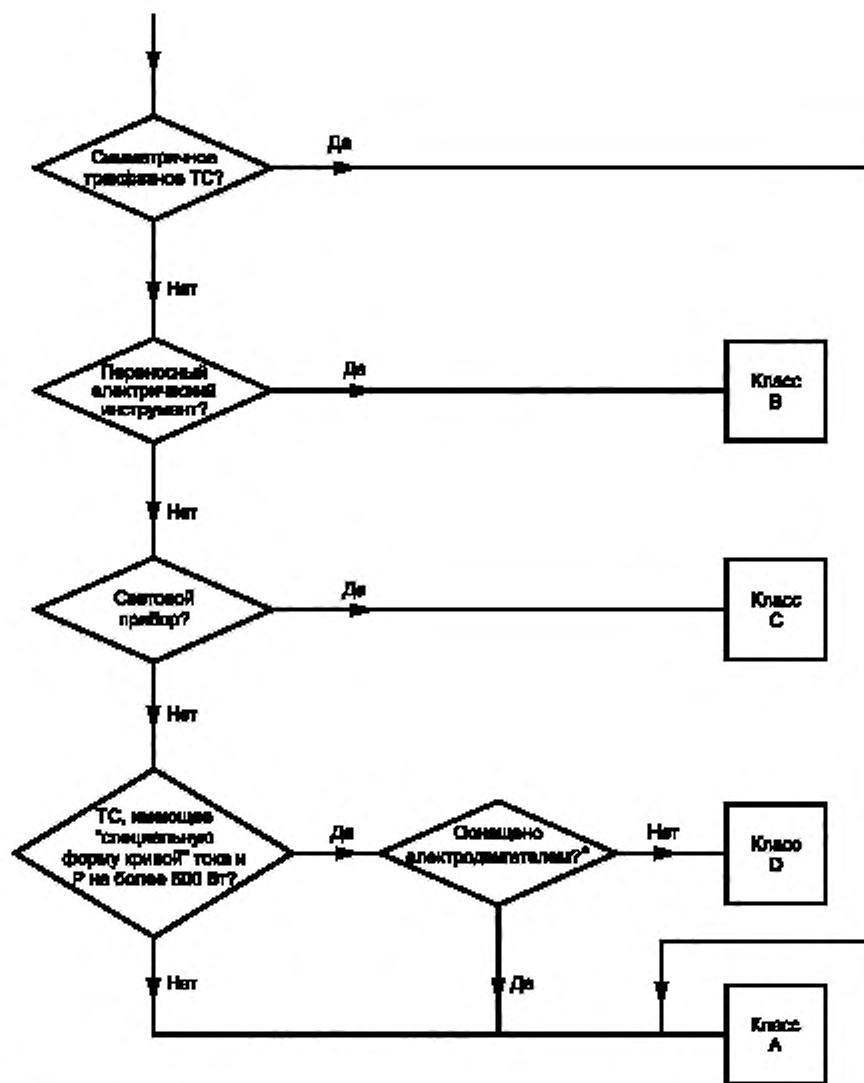
Рисунок 2 — Алгоритм классификации ТС
