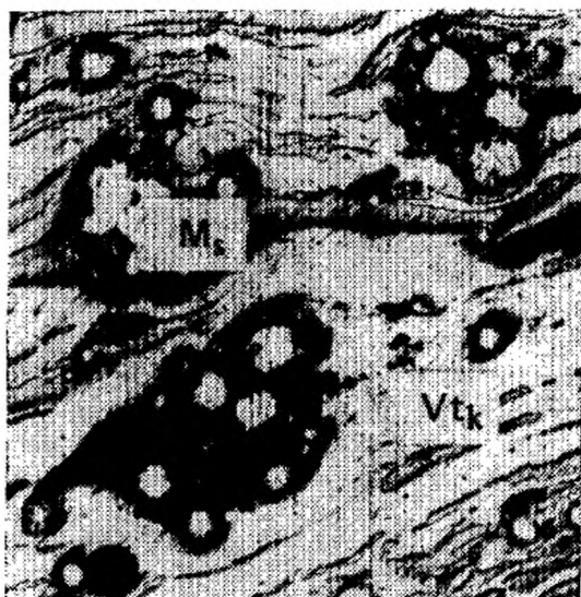
Vt_k — коллинит; M_s — сульфиды железа
