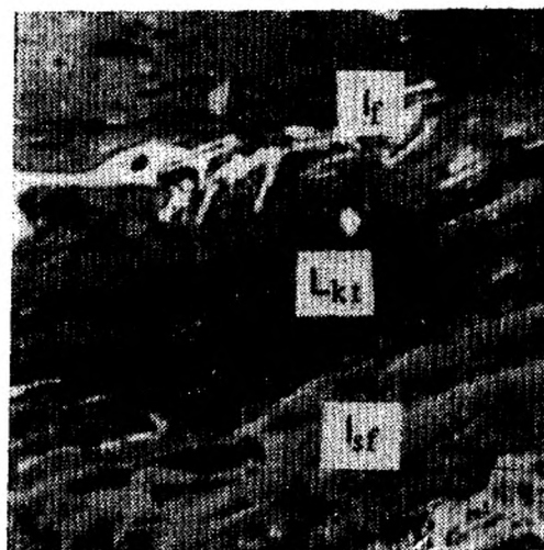
L_{kt} — кутинит; I_{sf} — семифузинит; I_f — фузинит
