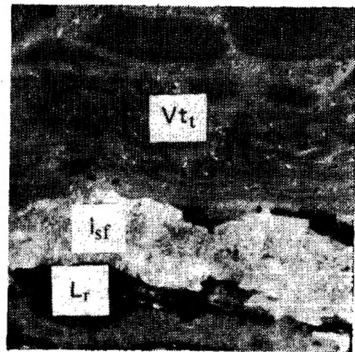
Vt_t — телинит; I_{sf} — semifюзинит; L_r — резинит
