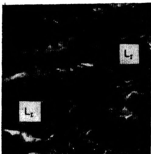
L_r — резинит Рисунок 11 — Масляная иммерсия 665×
