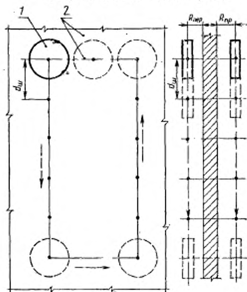
1 — рамочная антенна, 2 — портал дверного проема
