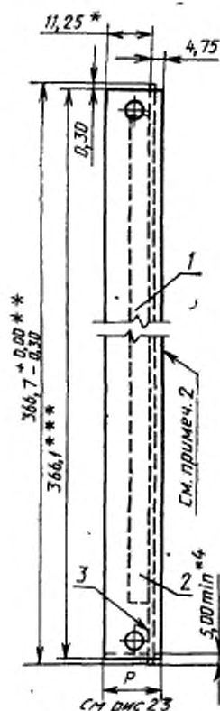
Рис. 29 Передняя панель на печатной плате модуля
