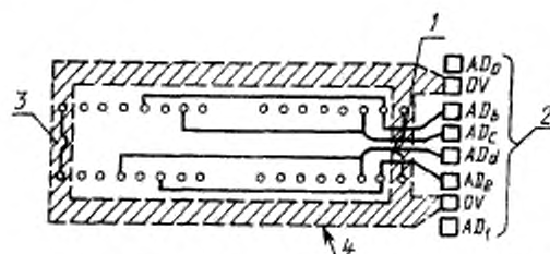
1 — типовая интегральная схема ЭСЛ 10К, используемая в качестве формирователя сигналов, подаваемых в шину; 2 — соединения с шиной; 3 — типовая интегральная схема ЭСЛ 10К, используемая в качестве приемника сигналов поступающих в шину; 4 — наилучшее исполнение или земляных проводников в виде плоской шины
