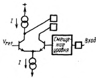
Рис. 38. Схематическое изображение формирователя для кабель-сегмента
