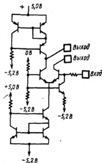
Рис. 39. Пример схемы формирователя для кабель-сегмента
