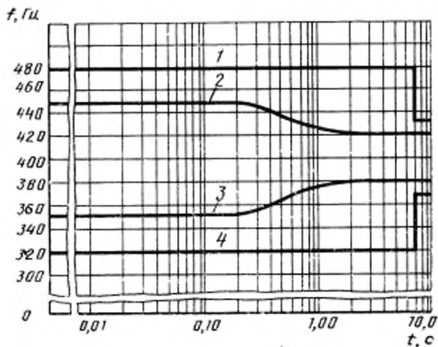
Пределы 1—4 значений переходной частоты
