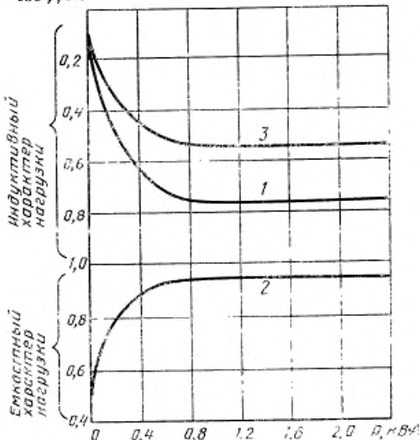
Пределы 1—3 значений коэффициента мощности приемников \cos \varphi, \text{ а. е.}
