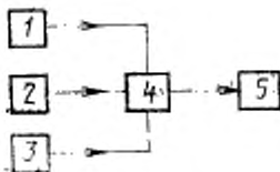
1—источник питающих напряжений электродов трубки; 2—блок формирования импульсов подсвета; 3—развертывающее устройство; 4—трубка; 5—прибор
