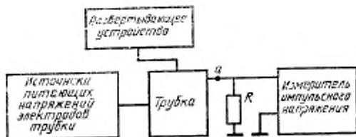
а—вывод электрода временной отклоняющей системы или экрана трубки; R—резистор
