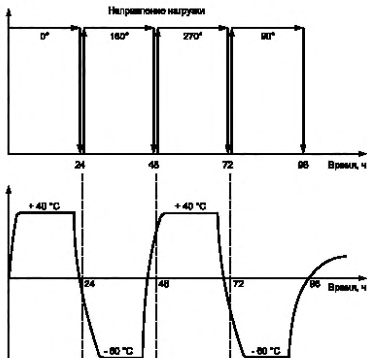
Рисунок 4 — Термомеханические испытания
