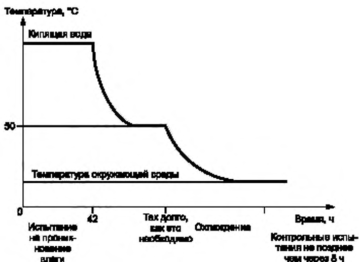
Рисунок 6 — Испытания на проникновение влаги
