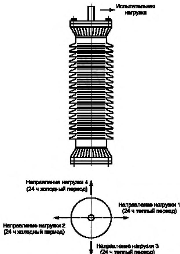
Рисунок 5 — Направления действия изгибающей нагрузки при термомеханических испытаниях
