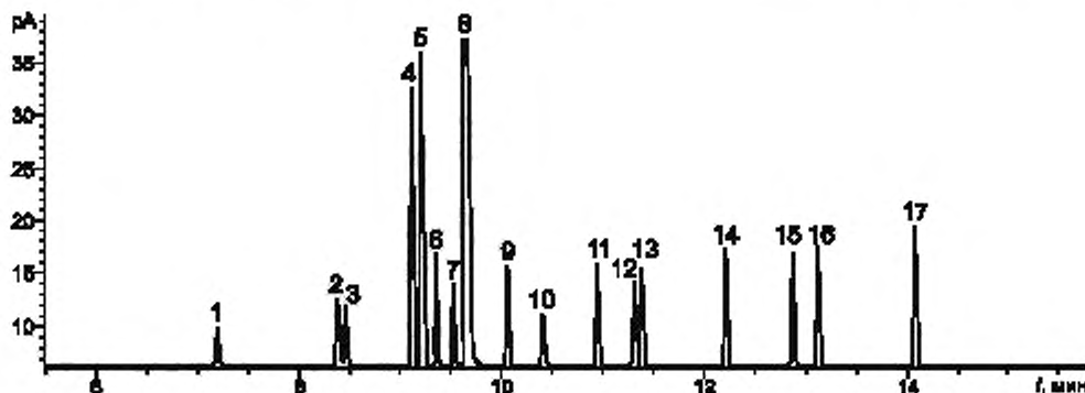
1 — уксусный альдегид; 2 — ацетон; 3 — этилформиат; 4 — этилацетат; 5 — метанол; 6 — 2-бутанол; 7 — 2-пропанол; 8 — этанол; 9 — этилпропионат; 10 — диацетил; 11 — изобутилацетат; 12 — 1-пропанол; 13 — этилбутират; 14 — изобутиловый спирт; 15 — изоамилацетат; 16 — 1-бутанол; 17 — изоамиловый спирт
