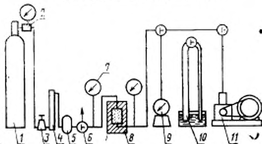
Принципиальная схема установки для определения газопроницаемости
