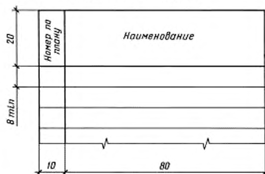
Экспликация помещений
