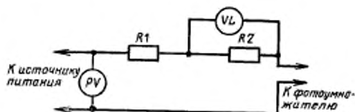
PV — вольтметр; R1, R2 — резисторы по ГОСТ 7113—77; VL — неоновая лампа.
